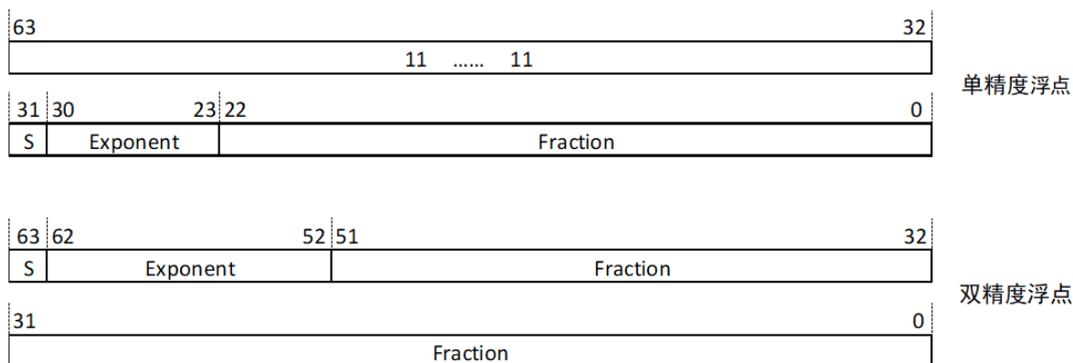
图 4.3: 浮点数据格式
