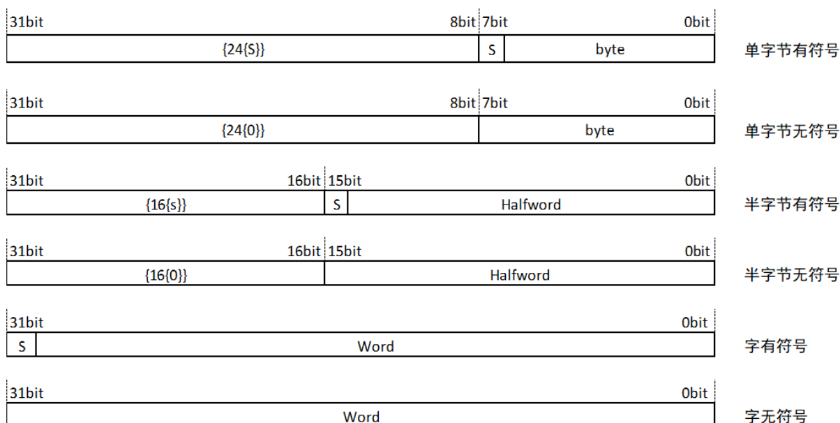
图 4.2: 寄存器中的整型数据组织结构
