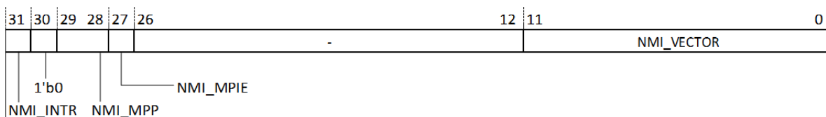
图 18.11: NMI 状态寄存器 (MNMICAUSE)
