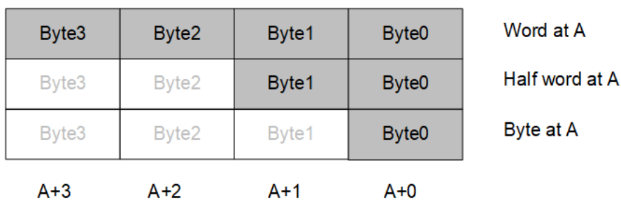
图 4.4: 内存中的数据组织形式
