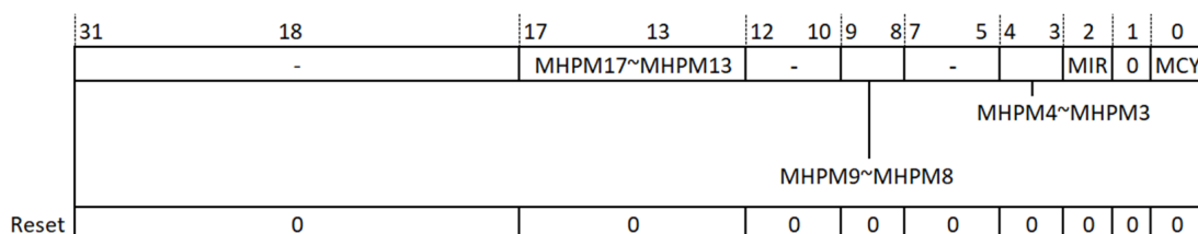
图 15.2: 机器模式计数禁止授权寄存器 (MCOUNTINHIBIT)
