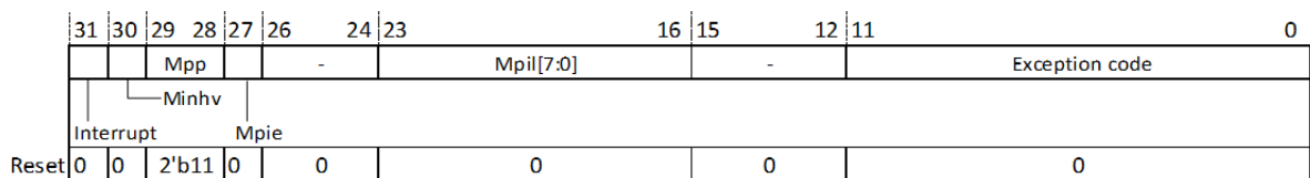
图 18.5: 机器模式异常事件向量寄存器 (MCAUSE)
