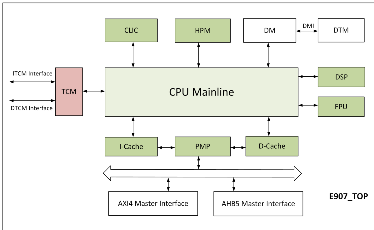
图 9.2: TCM 接口
