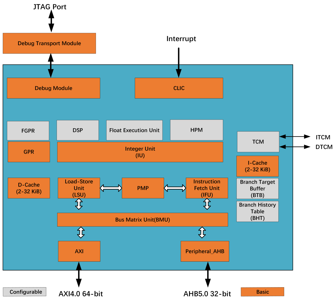
图 2.1: E907 结构图
