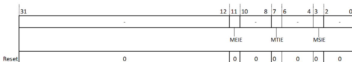
图 18.2: 机器模式中断使能控制寄存器（MIE）
