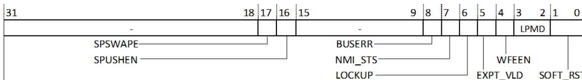
图 18.10: 扩展异常状态寄存器 (MEXSTATUS)
