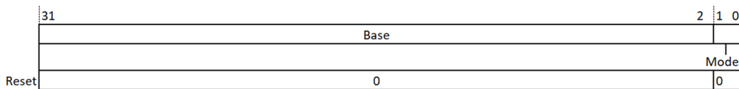
图 18.3: 机器模式异常向量基址寄存器 (MTVEC)
