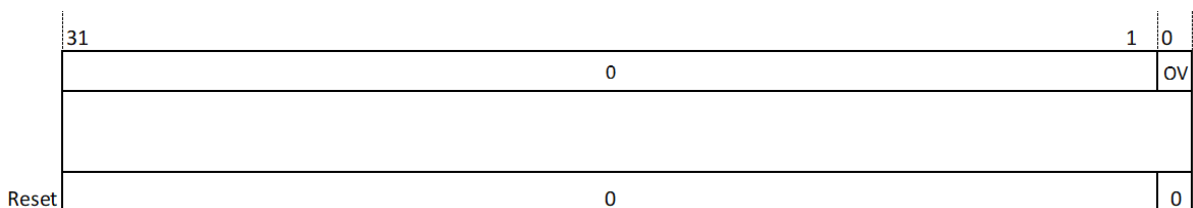
图 18.16: 定点运算饱和状态寄存器 (VXSAT)
