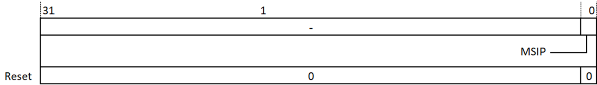
图 7.1: 机器模式软件中断配置寄存器 (MSIP)
