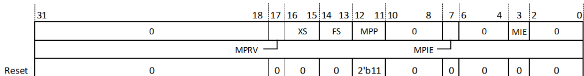
图 18.1: 机器模式处理器状态寄存器 (MSTATUS)
