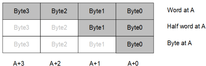
图 3.4: 内存中的数据组织形式
