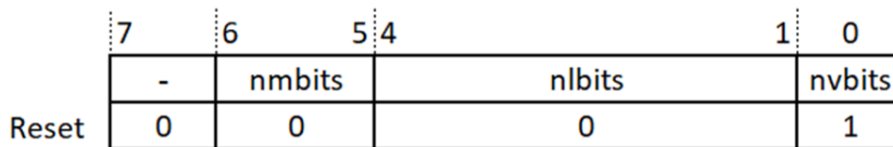
图 10.1: CLIC 配置寄存器 (CLICCFG)
