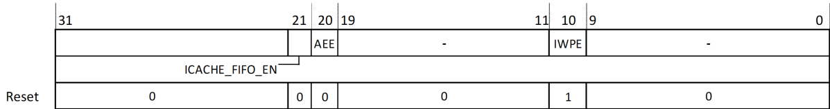
图 17.9: 隐式操作寄存器 (MHINT)
