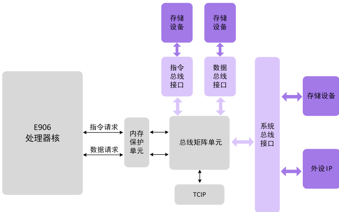
图 8.1: E906 总线矩阵
