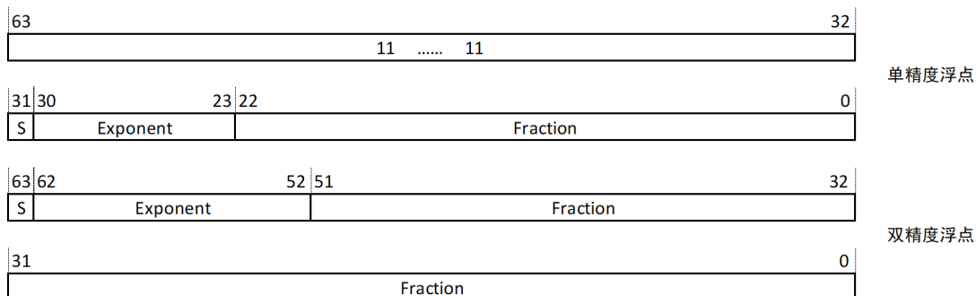
图 3.3: 浮点数据格式
