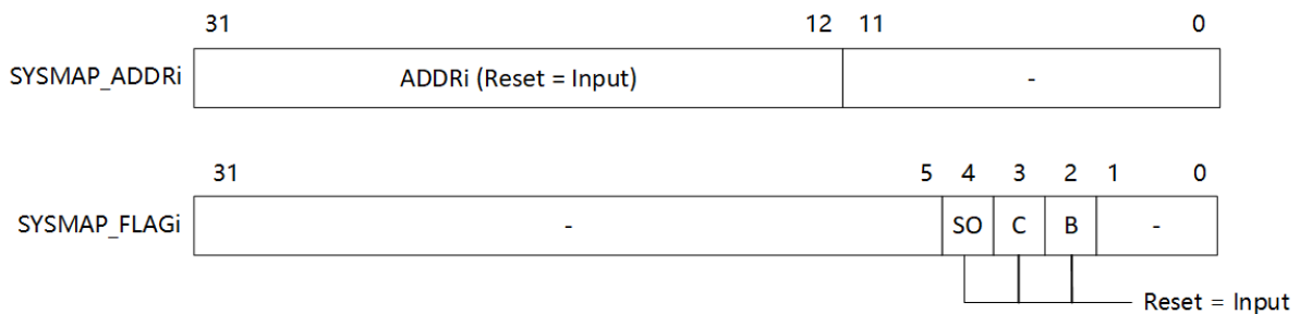
图 7.2: SYSMAP 寄存器的格式
