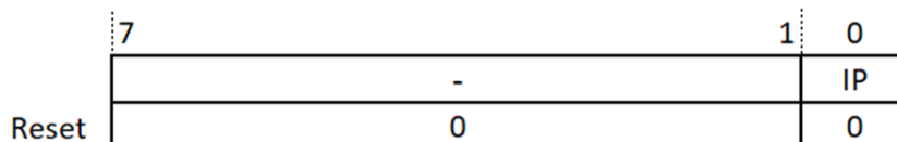
图 10.4: 中断等待寄存器 (CLICINTIP)
