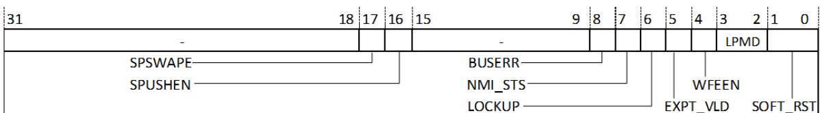
图 17.10: 扩展异常状态寄存器 (MEXSTATUS)
