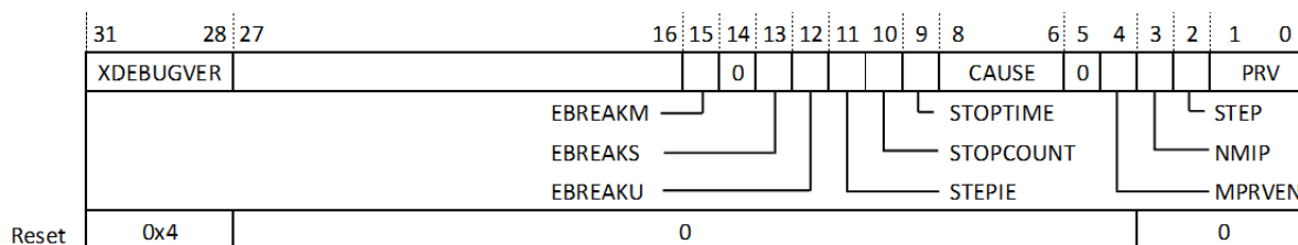
图 17.20: 调试模式控制与状态寄存器 (DCSR)
