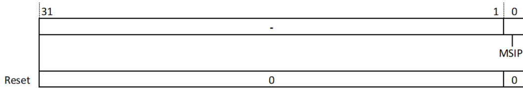
图 9.1: 机器模式软件中断配置寄存器 (MSIP)
