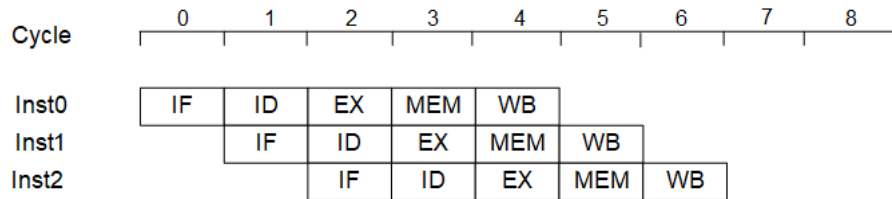
图 2.2: 单周期指令执行过程
