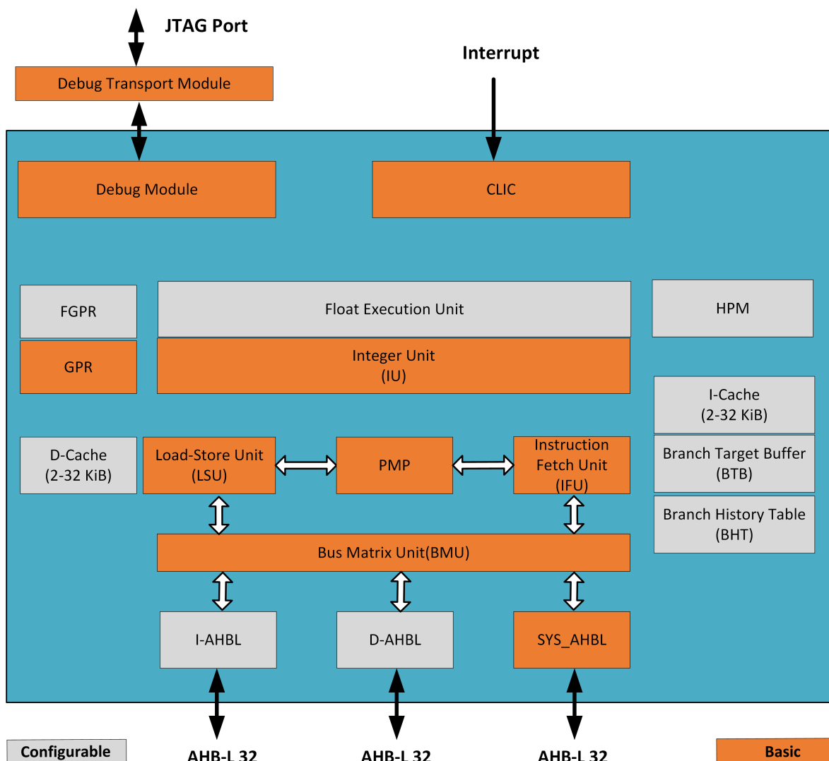
图 2.1: E906 结构图
