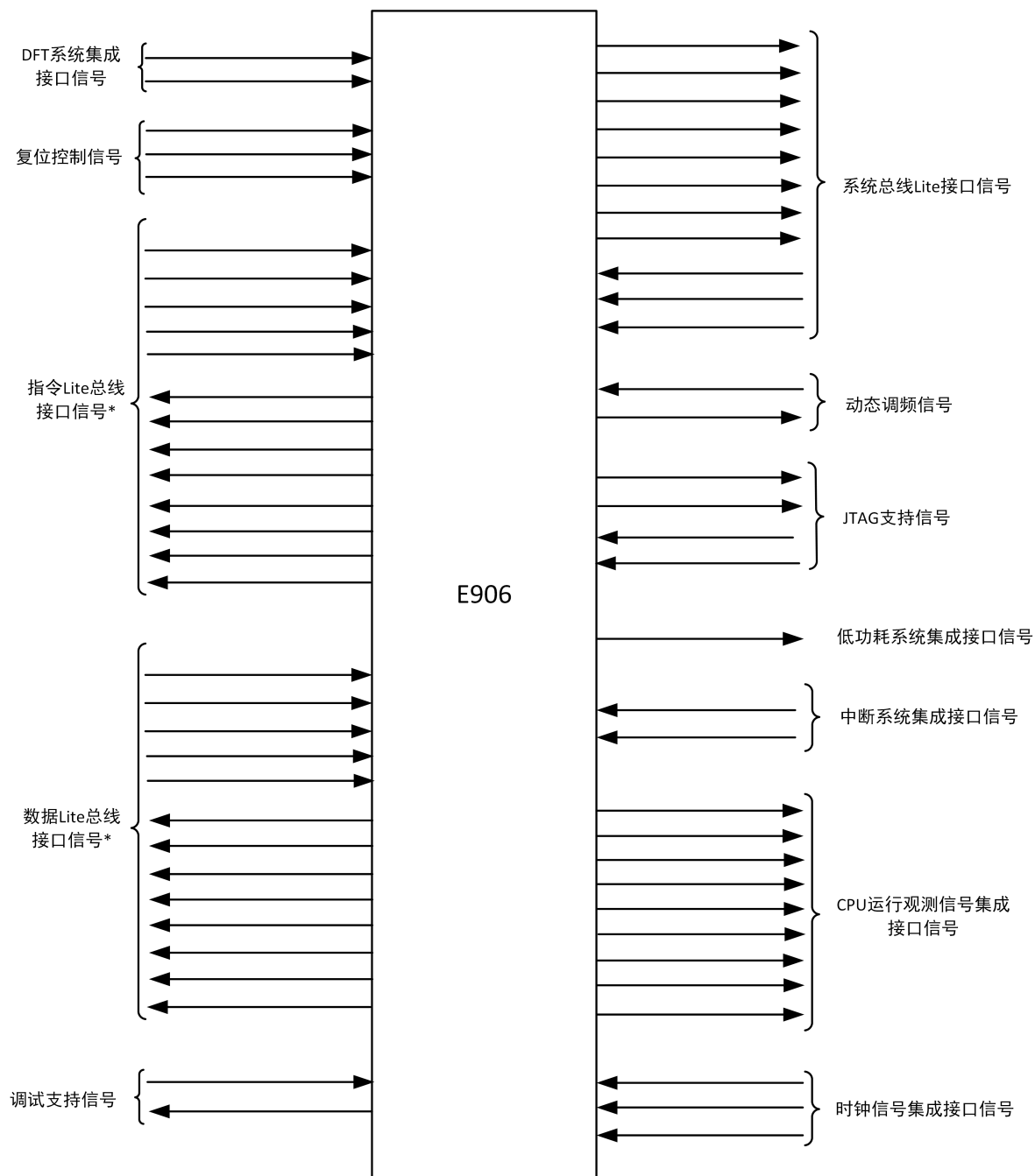
图 2.7: E906 接口总览
