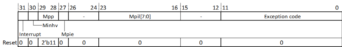
图 16.5: 机器模式异常事件向量寄存器 (MCAUSE)
