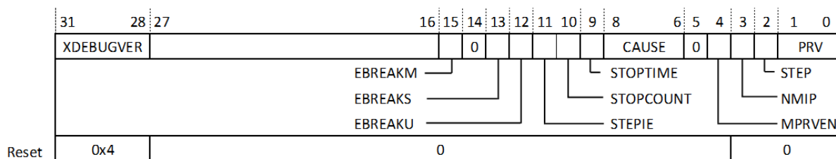
图 16.20: 调试模式控制与状态寄存器 (DCSR)
