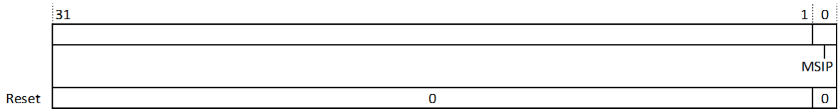
图 9.1: 机器模式软件中断配置寄存器 (MSIP)
