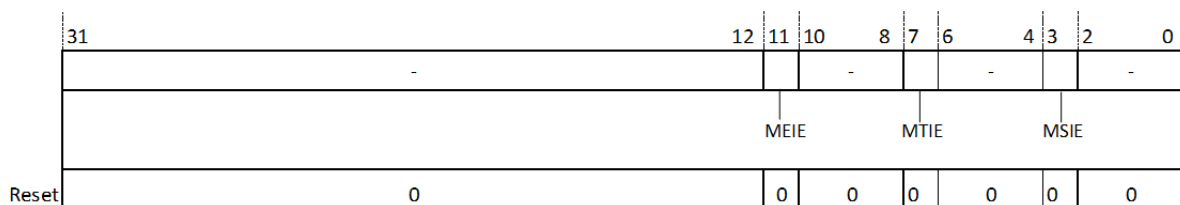
图 16.2: 机器模式中断使能控制寄存器 (MIE)
