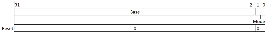
图 16.3: 机器模式异常向量基址寄存器 (MTVEC)
