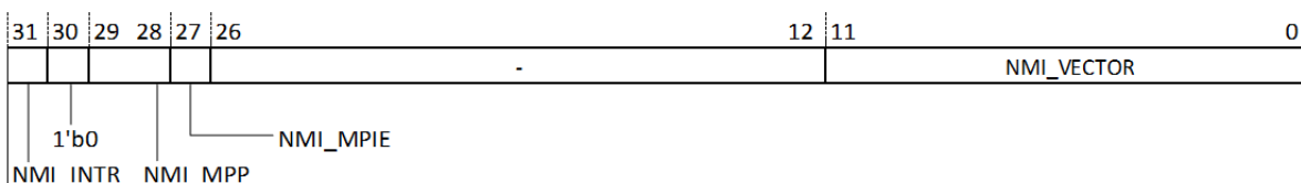
图 16.11: NMI 状态寄存器 (MNMICAUSE)
