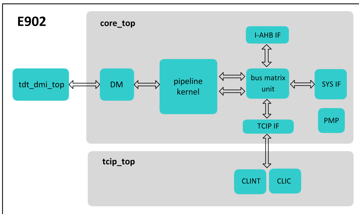
图 2.1: E902 结构图
