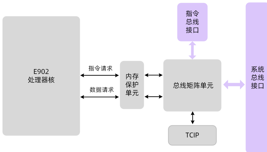
图 8.1: E902 总线矩阵
