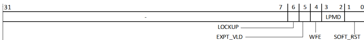
图 16.10: 扩展异常状态寄存器 (MEXSTATUS)
