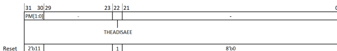
图 16.7: 扩展状态寄存器 (MXSTATUS)
