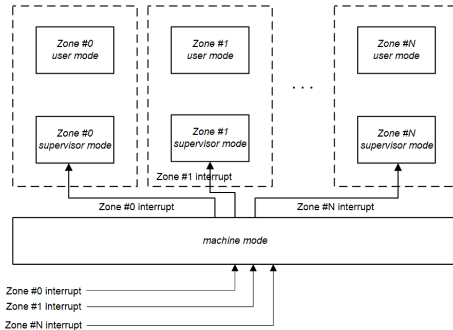
图 9.8: 玄铁 RISC-V 处理器 M 模式中中断分发
