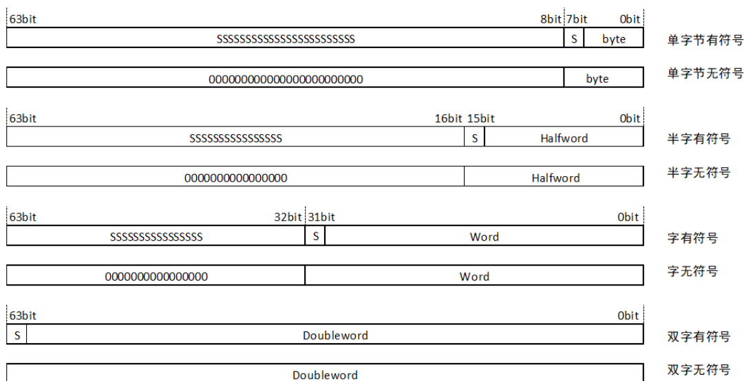
图 4.2: 寄存器中的整型数据组织结构
