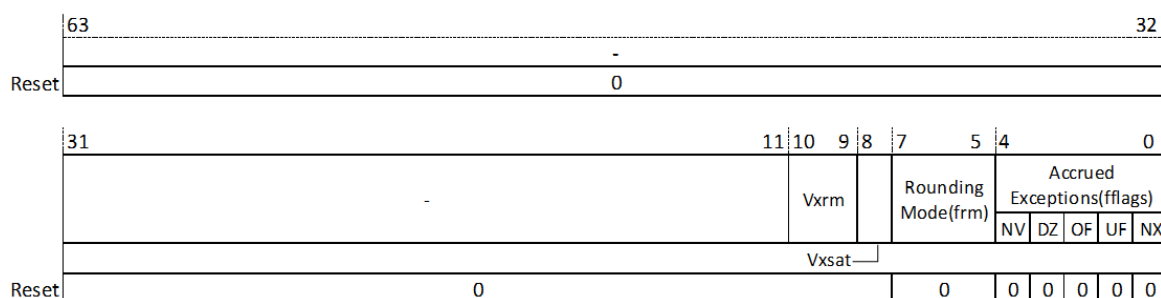
图 18.29: 浮点控制状态寄存器 (FCSR)
