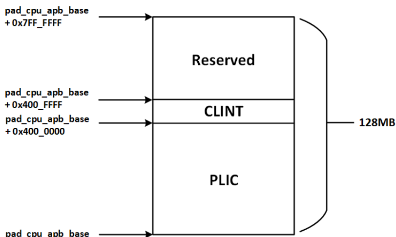
图 10.5: PLIC&CLINT 地址空间
