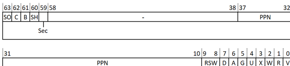
图 6.7: SMEL 寄存器说明
