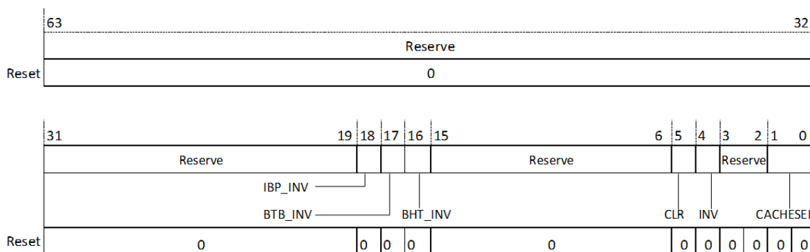
图 18.9: 机器模式硬件操作寄存器 (MCOR)
