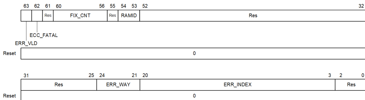
图 18.11: 机器模式 L2Cache ECC 控制寄存器 (MCER2)
