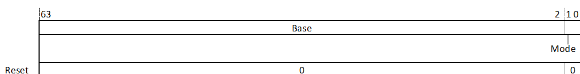
图 18.27: 超级用户模式向量基址寄存器 (STVEC)
