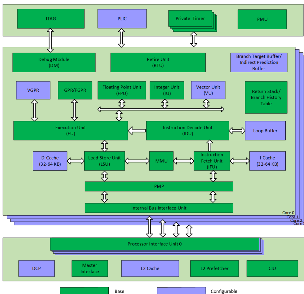
图 2.1: C910/C920MP 微体系结构图 (C910 不含 Vector Unit)
