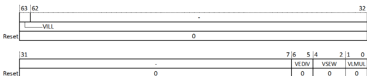
图 18.32: 矢量数据类型寄存器 (VTYPE)
