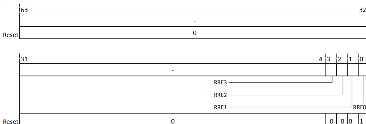
图 18.14: 机器模式复位寄存器 (MRMR)
