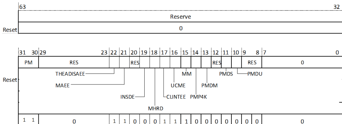
图 18.7: 机器模式扩展状态寄存器 (MXSTATUS)
