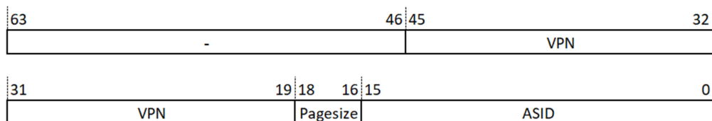
图 6.6: SMEH 寄存器说明
