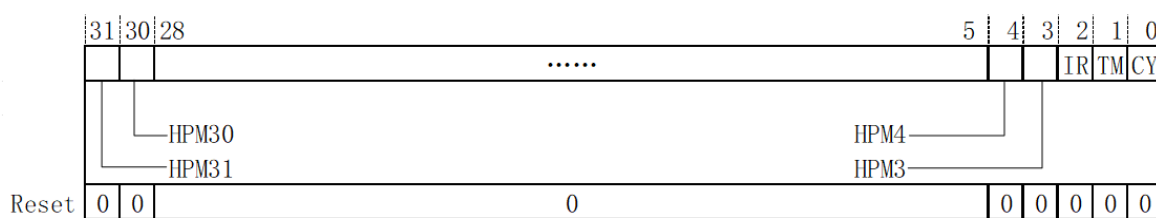
图 14.2: 超级用户模式计数器访问授权寄存器 (SCOUNTEREN)
