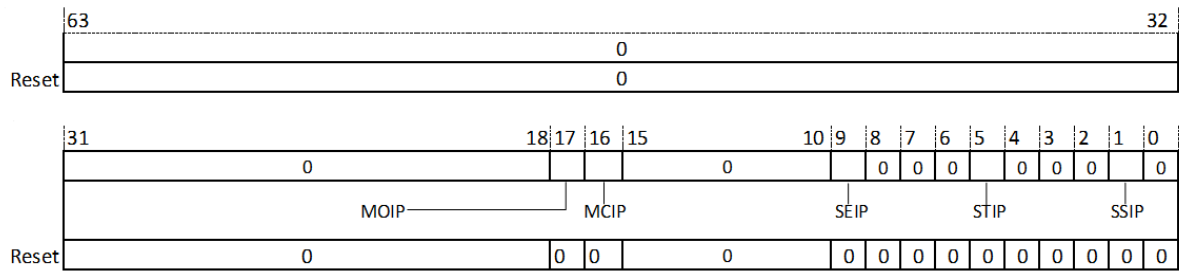
图 18.28: 超级用户模式中中断等待状态寄存器 (SIP)
