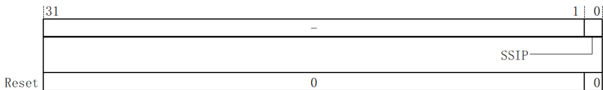
图 10.2: 超级用户模式软件中断配置寄存器 (SSIP)
