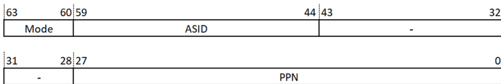
图 6.3: SATP 寄存器说明
