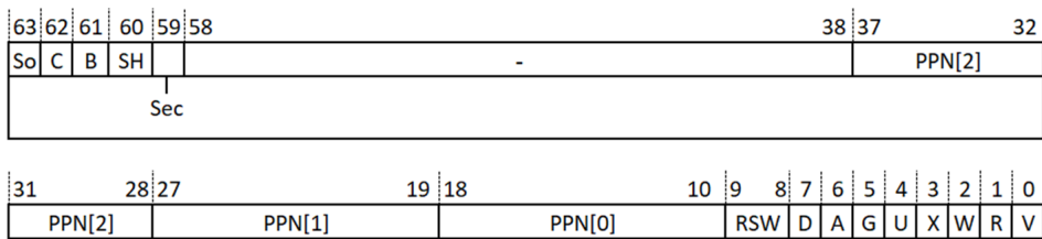
图 6.2: 页表结构说明
