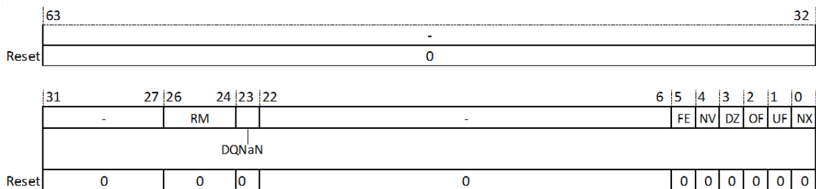
图 18.30: 浮点扩展控制寄存器 (FXCR)
