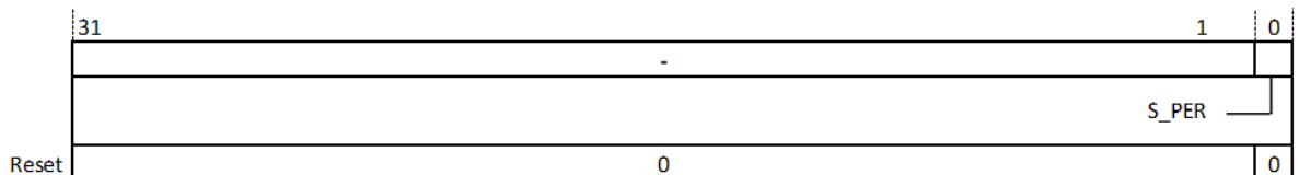
图 10.9: PLIC 权限控制寄存器 (PLIC_CTRL)
