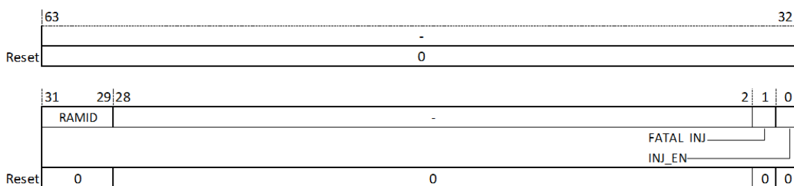
图 18.20: 机器模式 L1Cache 硬件错误注入寄存器 (MEICR)
