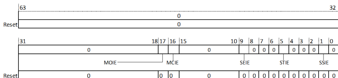
图 18.26: 超级用户模式中断使能控制寄存器 (SIE)
