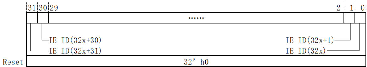
图 10.8: PLIC_IEx 中断使能寄存器 (PLIC_IE)
