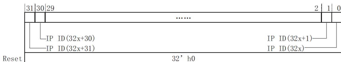
图 10.7: PLIC_IP x 中断等待寄存器 (PLIC_IP)
