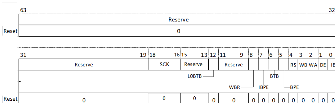
图 18.8: 机器模式硬件配置寄存器（MHCR）
