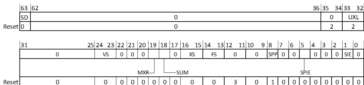
图 18.25: 超级用户模式处理器状态寄存器 (SSTATUS)
