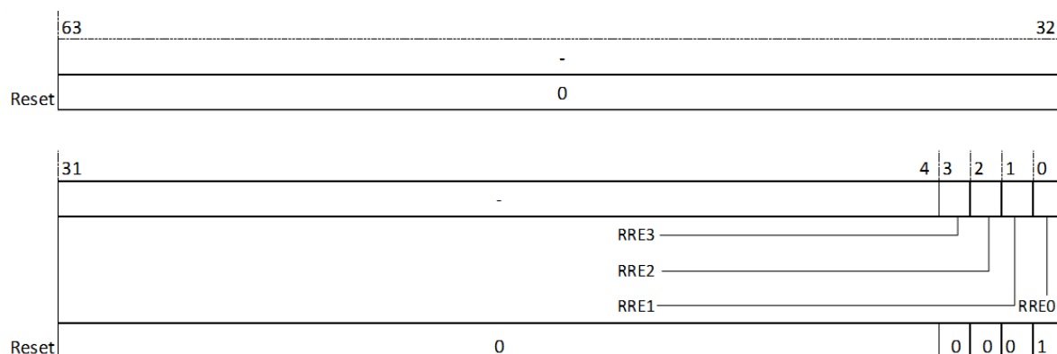
图 18.13: 机器模式复位寄存器 (MRMR)
