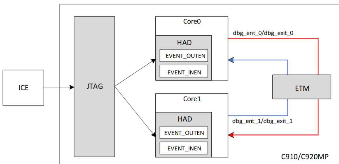
图 12.2: 多核调试整体框架
