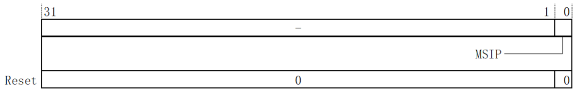
图 10.1: 机器模式软件中断配置寄存器 (MSIP)
