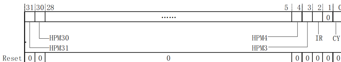
图 14.3: 机器模式计数禁止授权寄存器 (MCOUNTINHIBIT)
