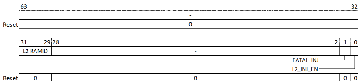
图 18.21: 机器模式 L2Cache 硬件错误注入寄存器 (MEICR2)
