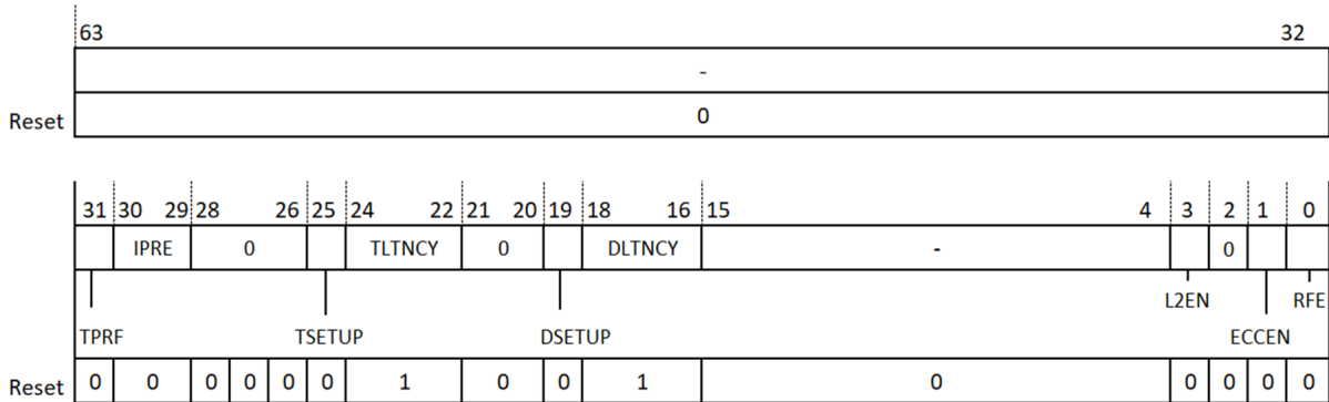
图 18.10: 机器模式 L2Cache 控制寄存器 (MCCR2)
