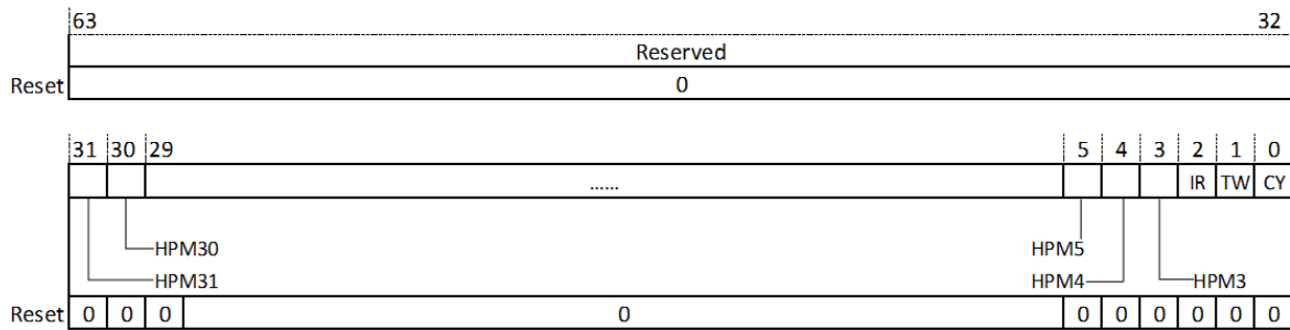
图 18.18: 机器模式事件中断使能寄存器 (MCOUNTERINTEN)
