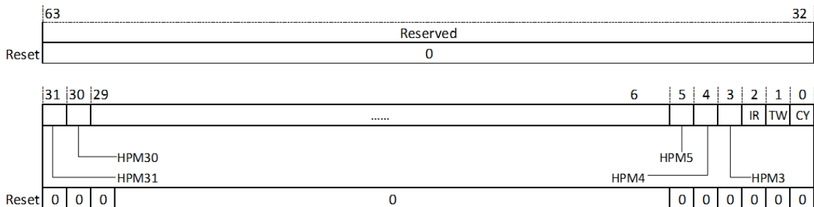
图 18.19: 机器模式事件上溢出标注寄存器 (MCOUNTEROF)
