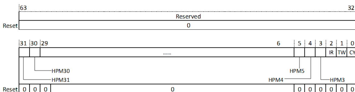
图 18.17: 机器模式计数器写使能寄存器 (MCOUNTERWEN)
