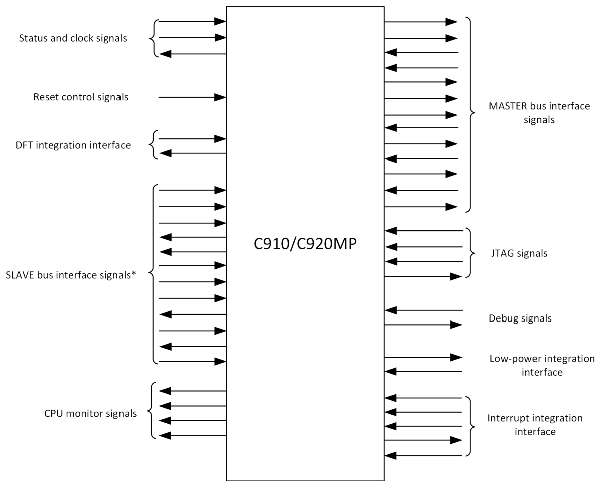
图 2.2: C910/C920 接口概览
