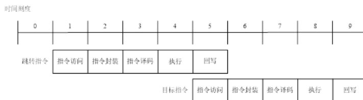
图 6.9: BT、BF、JSR、JMP 指令预测不正确时的执行过程
