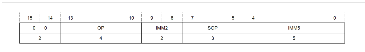
图 5.17: 七位立即数寻址方式
