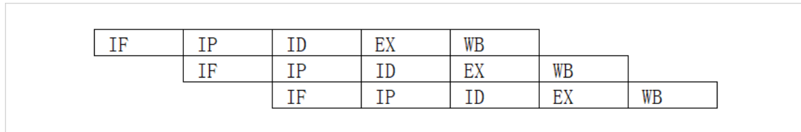
图 6.2: 单周期指令流水线重叠执行
