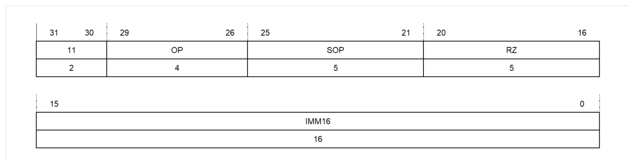
图 4.10: 一元寄存器十六位立即数寻址方式第二种格式
