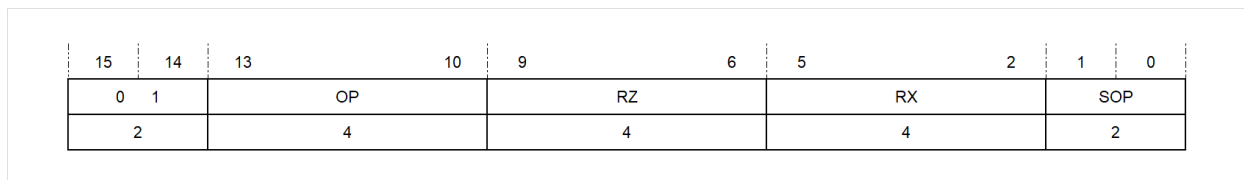
图 5.24: 二元寄存器寻址模式第三种格式
