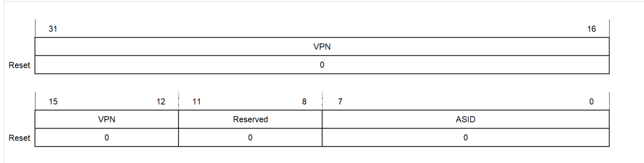
图 3.13: MMU EntryHi/Bad VPN 寄存器
