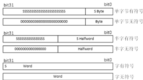
图 1.3: 寄存器中的数据组织结构
