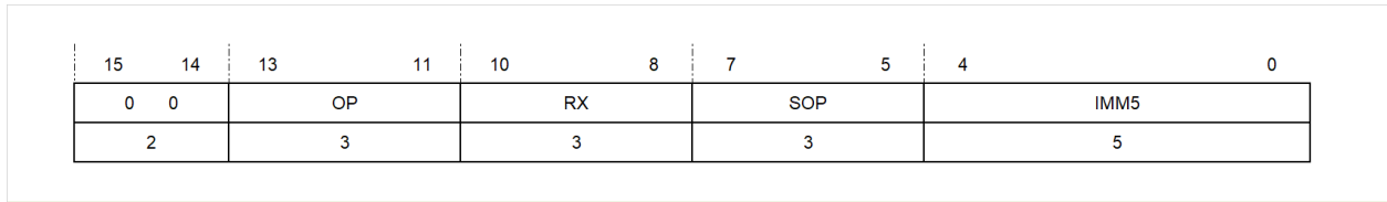
图 5.15: 一元寄存器五位立即数寻址方式
