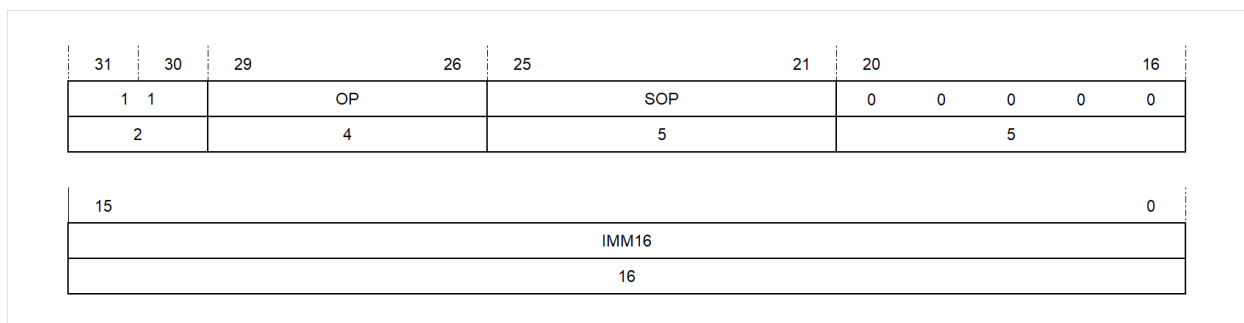
图 4.11: 十六位立即数寻址方式
