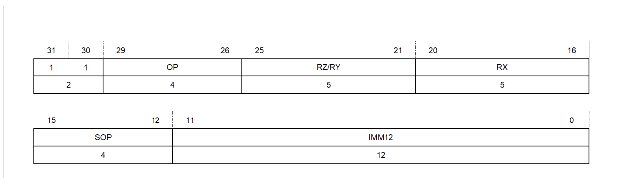
图 4.4: 12 位立即数的编码方式
