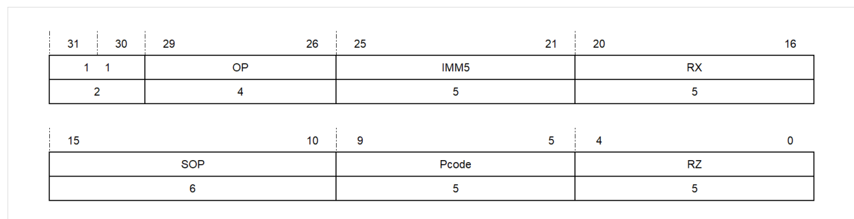
图 4.14: 二元寄存器五位立即数寻址方式第一种格式
