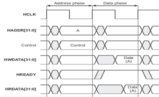
图 9.1: 简单传输
