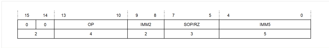
图 5.6: 7 位立即数的编码方式
