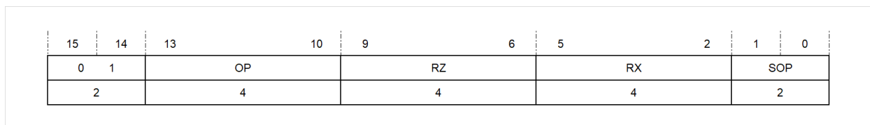
图 5.23: 二元寄存器寻址模式第二种格式
