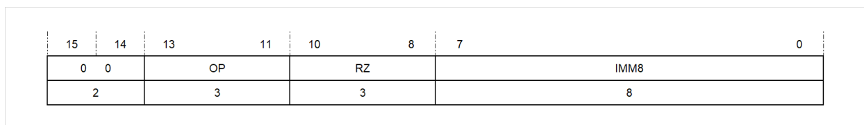
图 5.18: 一元寄存器八位立即数寻址方式第一种格式
