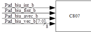
图 7.1: 中断接口信号
