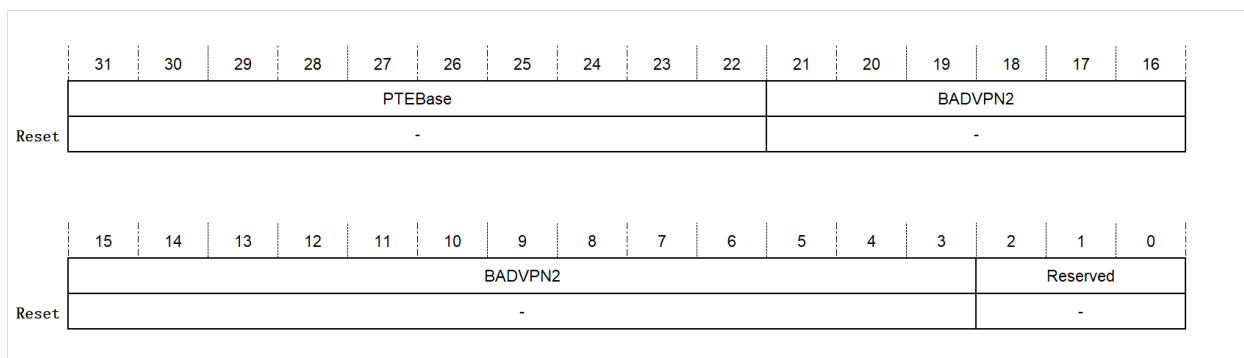
图 3.14: MMU 上下文寄存器
