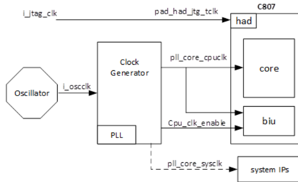
图 8.1: C807 的同步时钟管理方式
