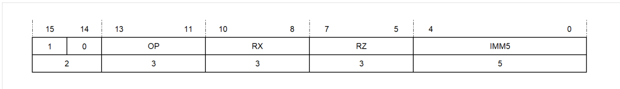
图 5.4: 5 位立即数的编码方式第二种格式
