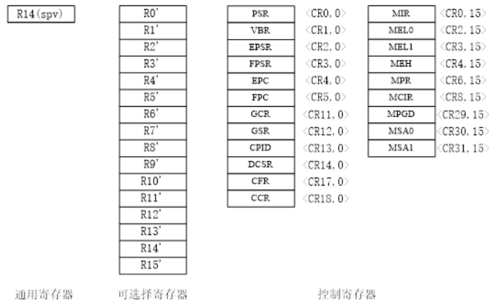
图 3.1: 超级用户编程模式附加资源
