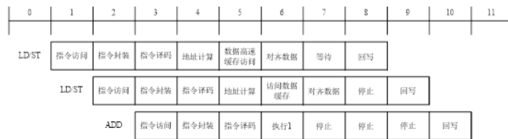
图 6.12: 带有等待状态的指令流水执行过程
