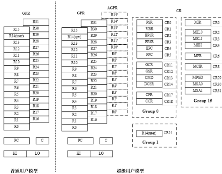
图 1.2: 编程模型
