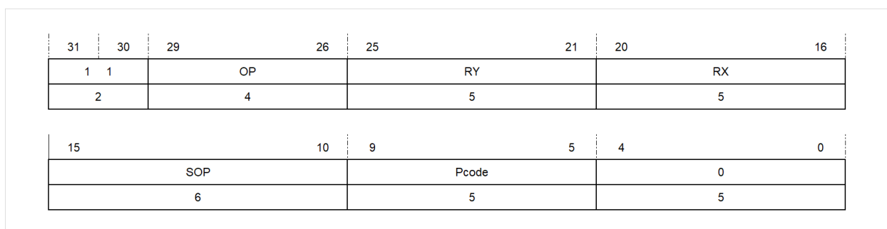
图 4.17: 二元寄存器寻址方式第二种格式
