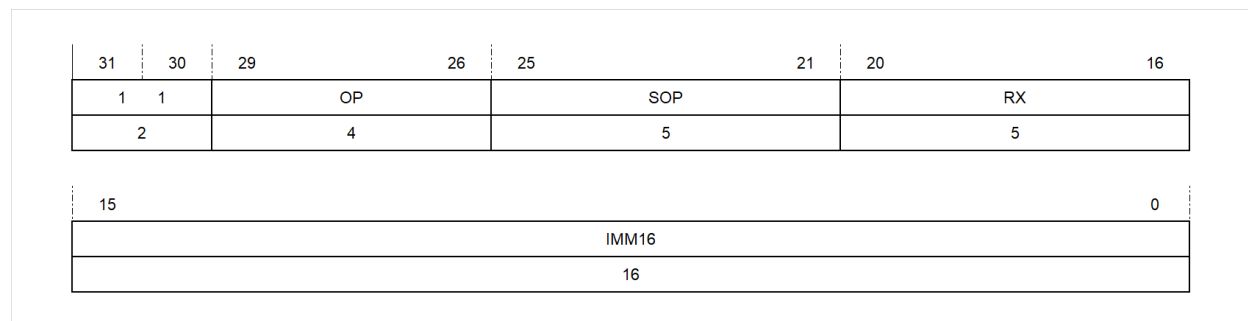
图 4.9: 一元寄存器十六位立即数寻址方式第一种格式
