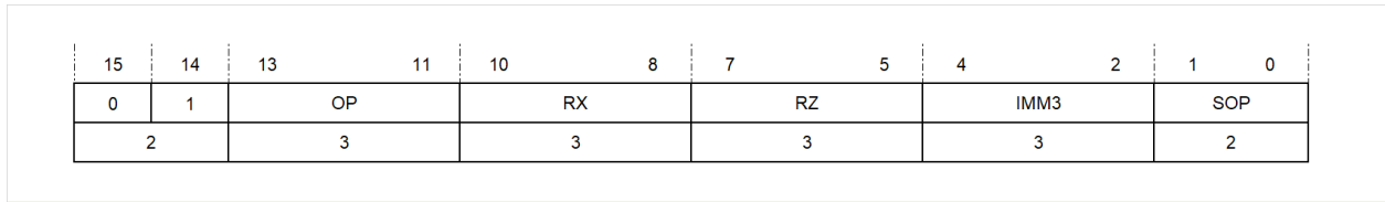
图 5.12: 二元寄存器三位立即数寻址方式
