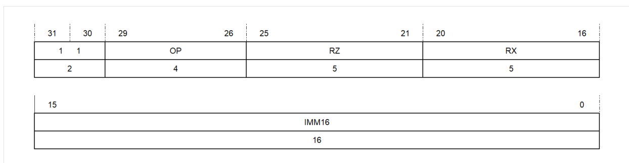
图 4.8: 二元寄存器十六位立即数寻址方式
