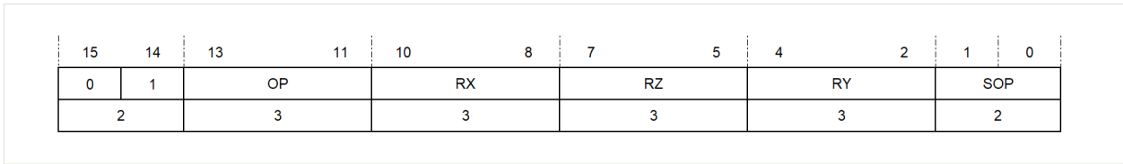
图 5.9: 3 操作数的编码方式
