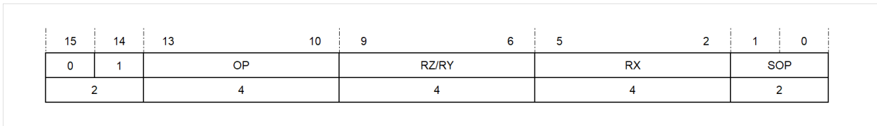
图 5.10: 2 操作数的编码方式
