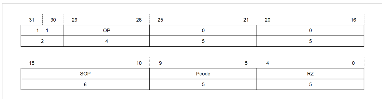
图 4.20: 一元寄存器寻址方式第一种格式
