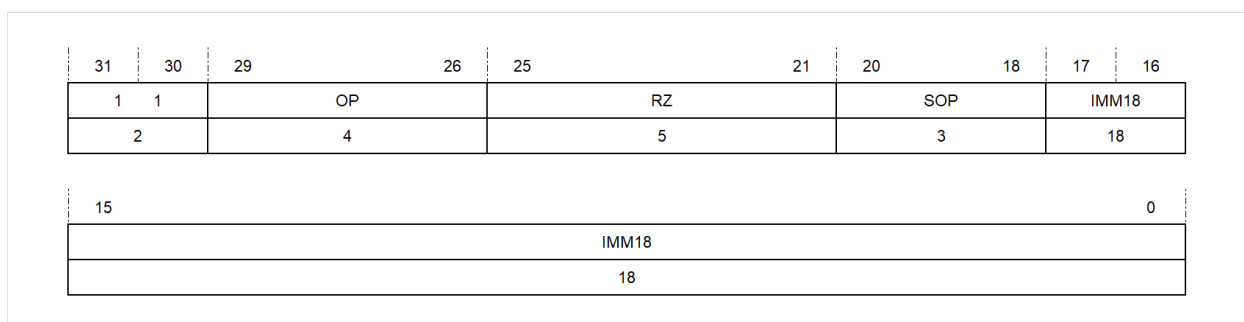
图 4.7: 一元寄存器十八位立即数寻址方式
