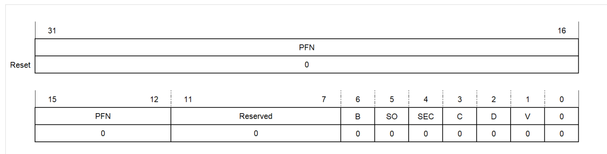
图 3.12: MMU EntryLo0 和 EntryLo1 寄存器
