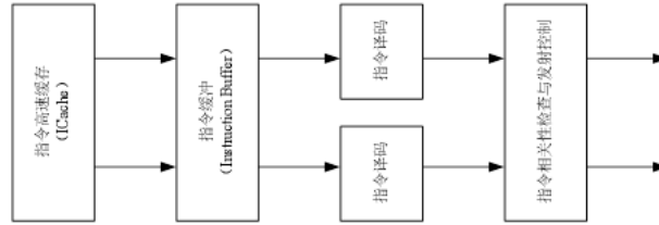
图 6.1: 指令执行时的数据流向
