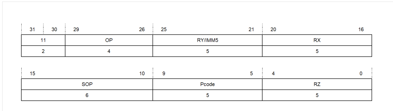
图 4.5: 寄存器类型
