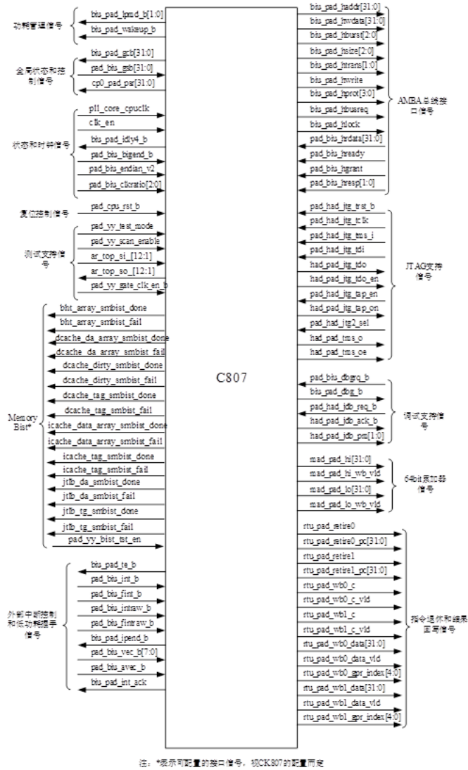
图 8.3: C807 顶层接口信号
