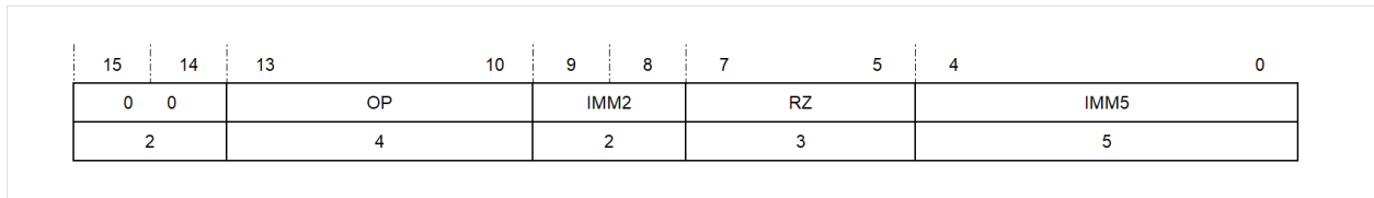
图 5.16: 一元寄存器七位立即数寻址方式
