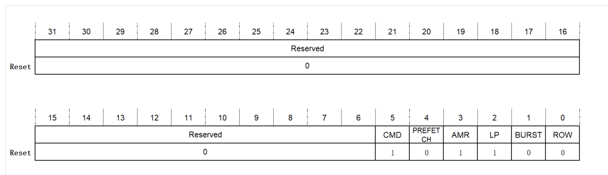
图 3.9: L2 高速缓存配置寄存器
