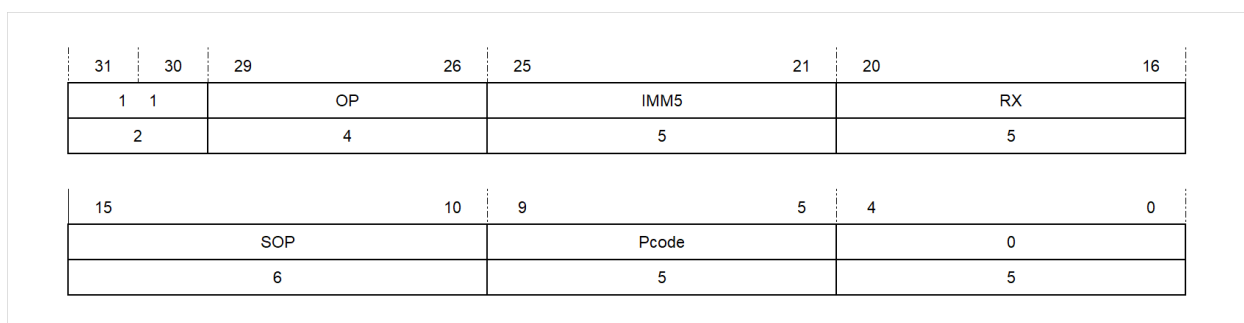
图 4.18: 一元寄存器五位立即数寻址方式第一种格式
