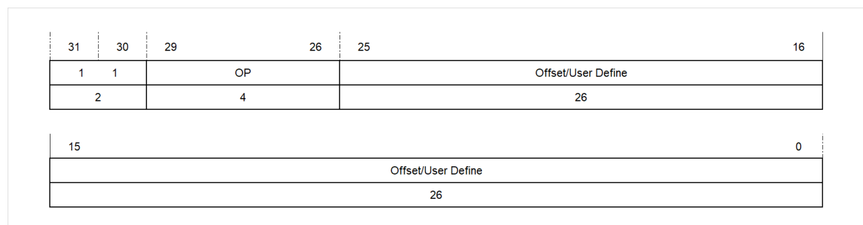
图 4.1: 跳转类型
