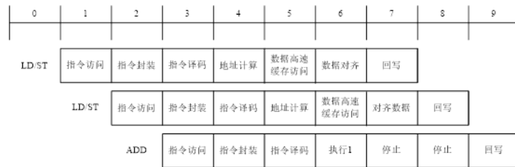
图 6.11: 简单的指令流水线执行过程
