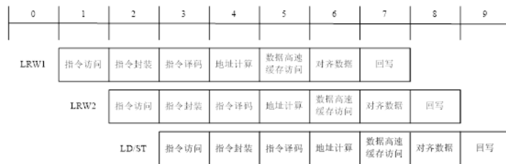
图 6.13: LRW 指令与访问存储指令混合的执行过程
