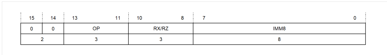
图 5.7: 8 位立即数的编码方式第一种格式
