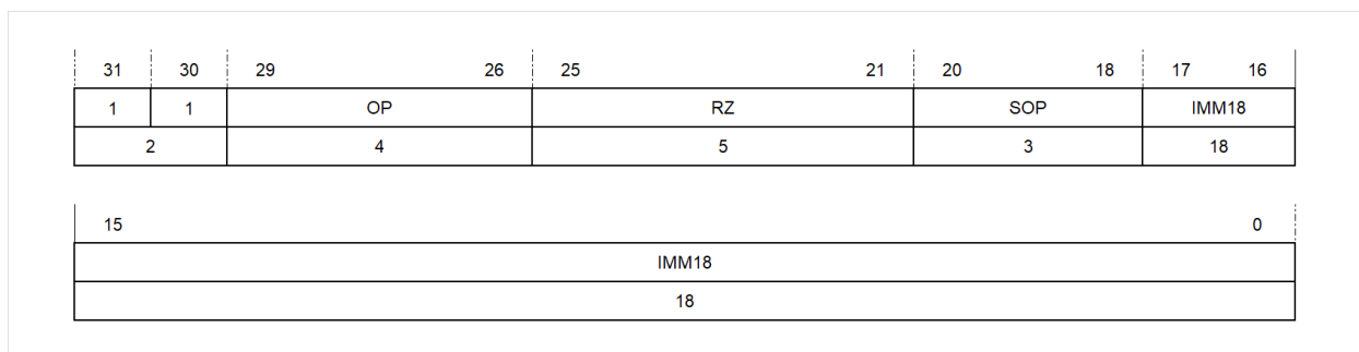
图 4.2: 18 位立即数的编码方式
