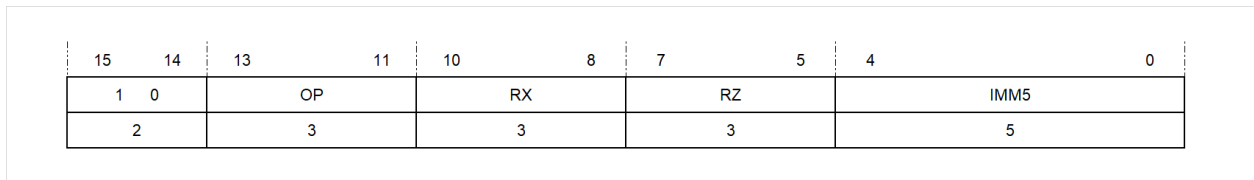
图 5.14: 二元寄存器五位立即数寻址方式第二种格式
