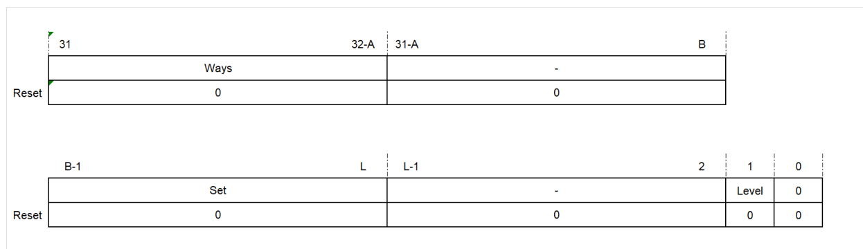
图 3.8: 高速缓存索引寄存器-2
