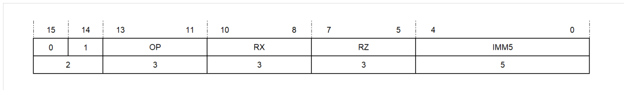
图 5.13: 二元寄存器五位立即数寻址方式第一种格式
