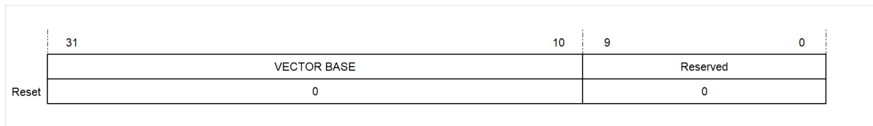
图 3.3: 基址向量寄存器
