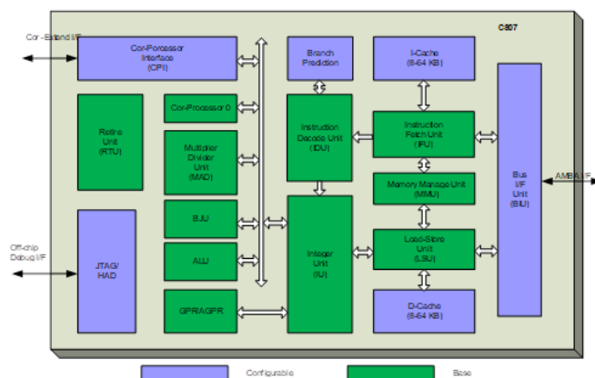
图 1.1: C807 结构图
