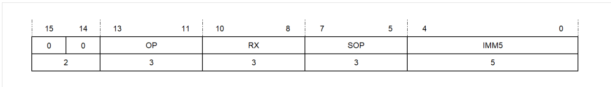
图 5.5: 5 位立即数的编码方式第三种格式
