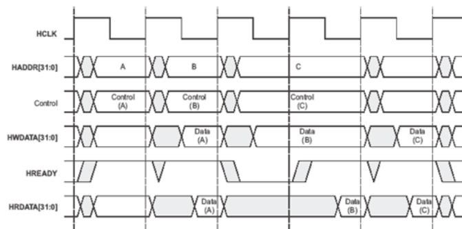
图 9.3: 多重传输
