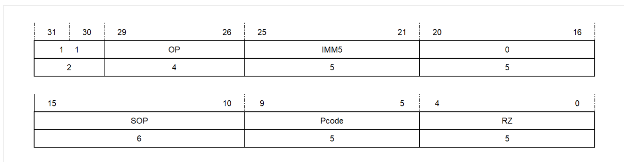
图 4.19: 一元寄存器五位立即数寻址方式第二种格式
