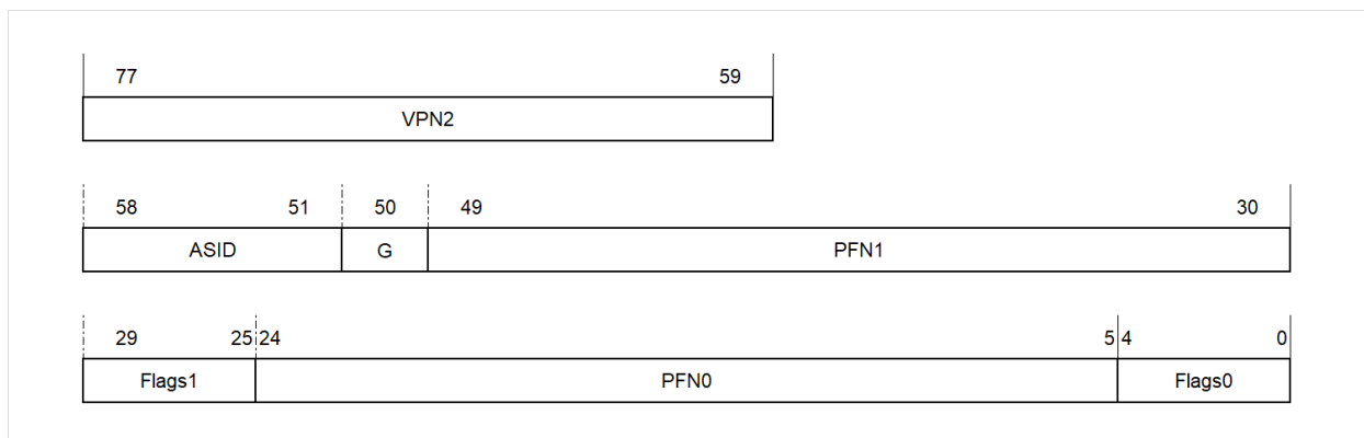
图 3.20: jTLB 表项
