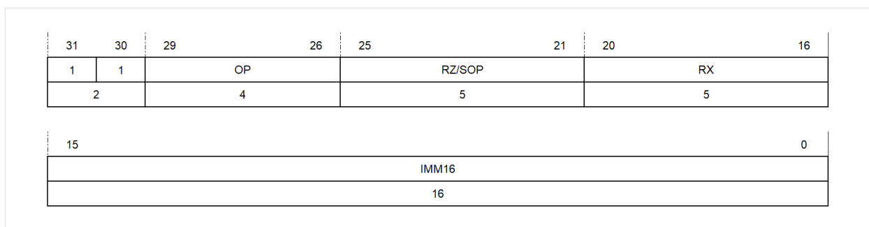
图 4.3: 16 位立即数的编码方式
