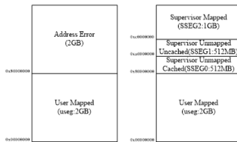
图 3.10: MMU 使用操作
