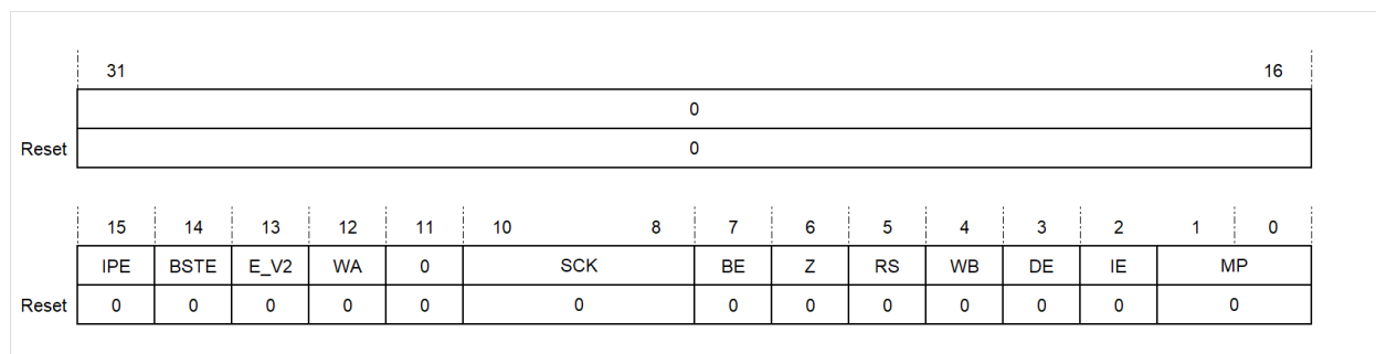
图 3.6: 高速缓存配置寄存器
