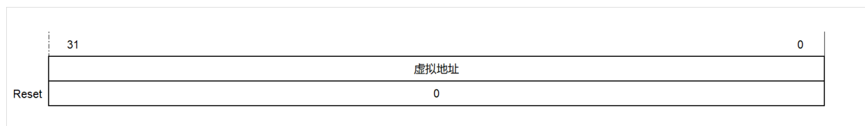
图 3.7: 高速缓存索引寄存器-1
