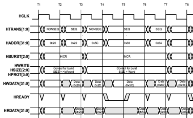
图 9.5: 增量突发传输
