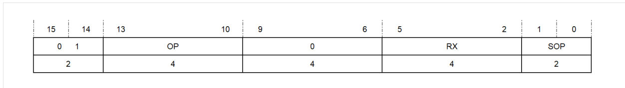
图 5.25: 一元寄存器寻址模式第一种格式
