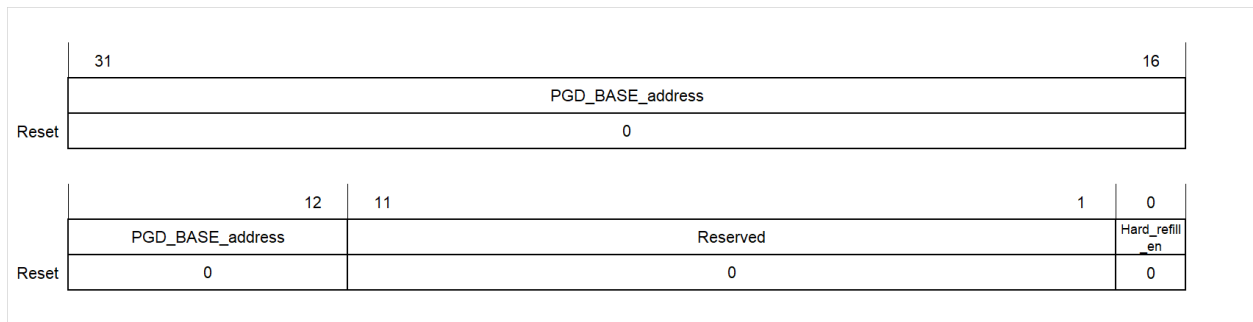
图 3.17: MMU PGD 基址寄存器
