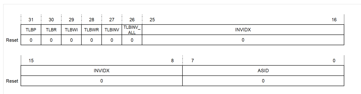
图 3.16: MMU 控制指令寄存器
