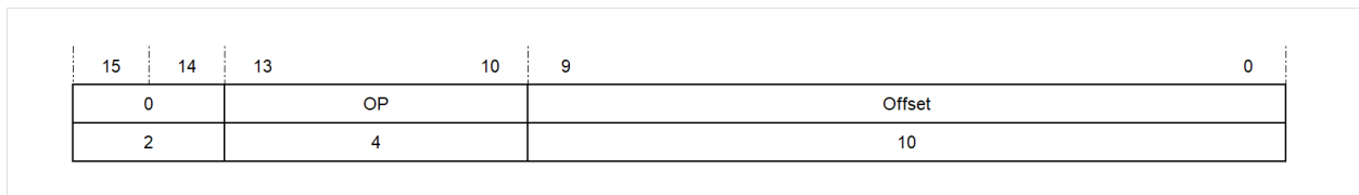
图 5.1: 跳转类型 (J 型)
