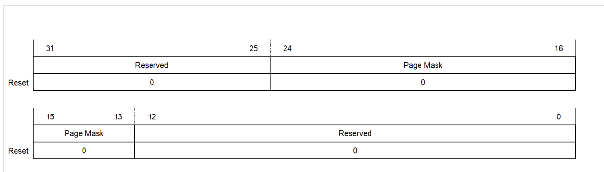
图 3.15: MMU 页掩码寄存器
