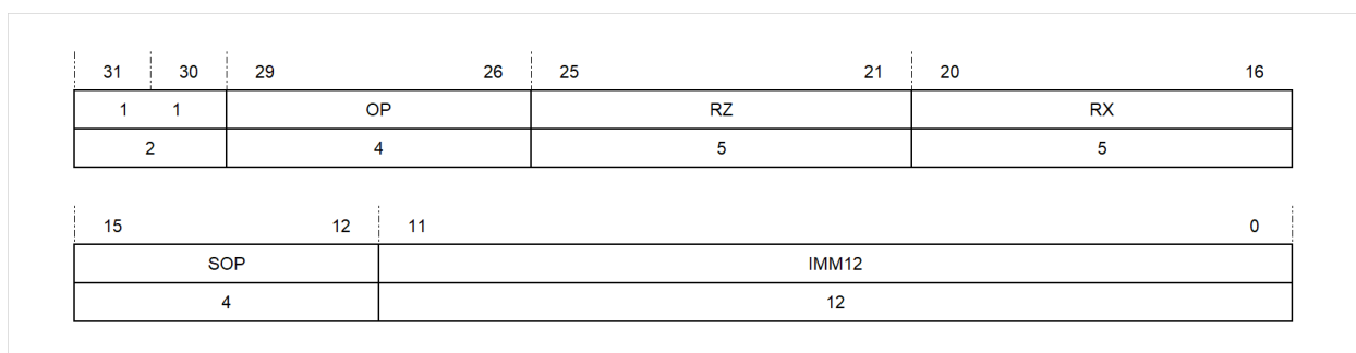
图 4.12: 二元寄存器十二位立即数寻址方式
