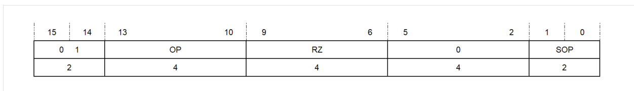
图 5.26: 一元寄存器寻址模式第二种格式
