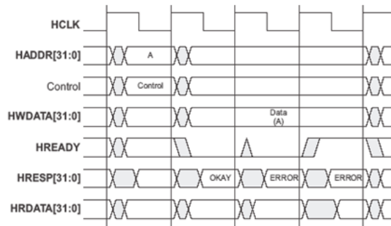
图 9.4: 错误响应
