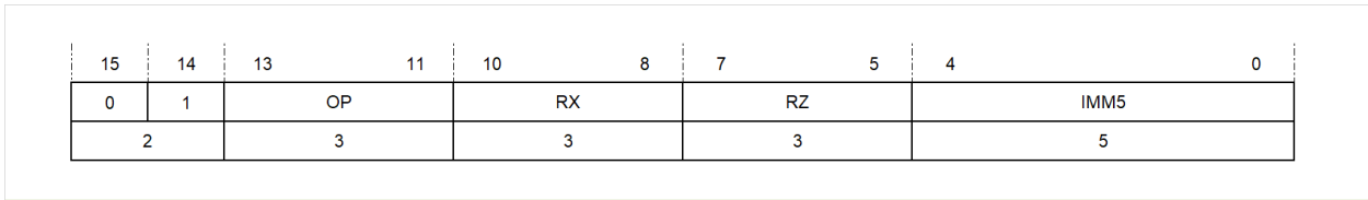
图 5.3: 5 位立即数的编码方式第一种格式
