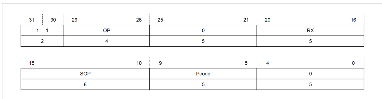
图 4.21: 一元寄存器寻址方式第二种格式
