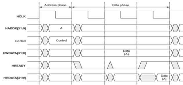
图 9.2: 有等待状态的传输
