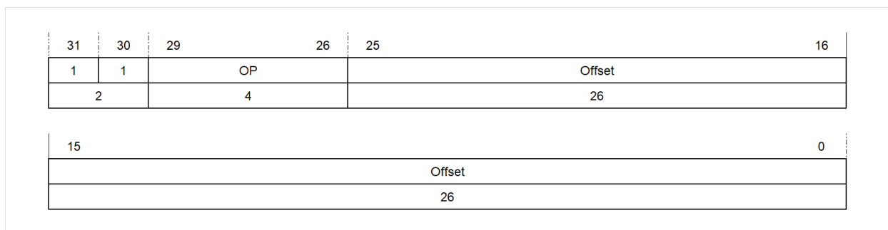
图 4.6: 二十六位立即数寻址方式
