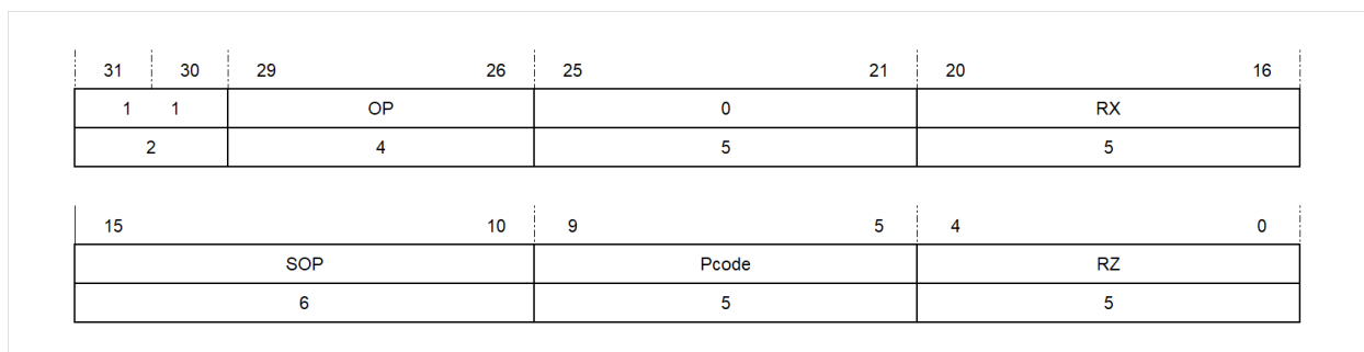
图 4.16: 二元寄存器寻址方式第一种格式
