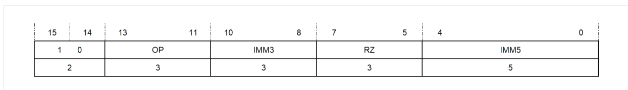
图 5.20: 一元寄存器八位立即数寻址方式第三种格式
