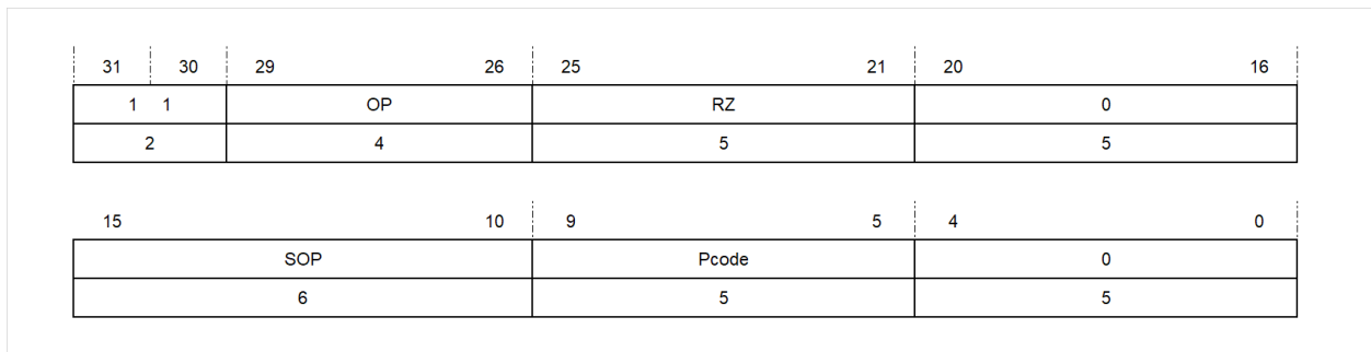
图 4.22: 一元寄存器寻址方式第三种格式
