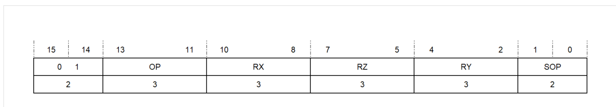
图 5.21: 三元寄存器寻址模式
