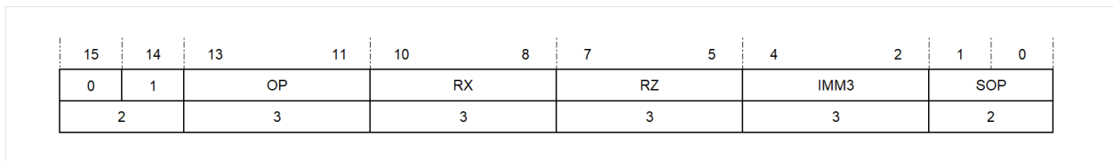
图 5.2: 3 位立即数的编码方式
