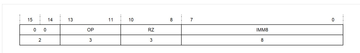
图 5.19: 一元寄存器八位立即数寻址方式第二种格式
