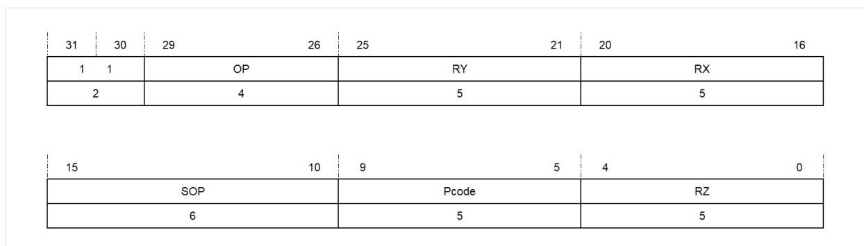
图 4.13: 三元寄存器寻址方式
