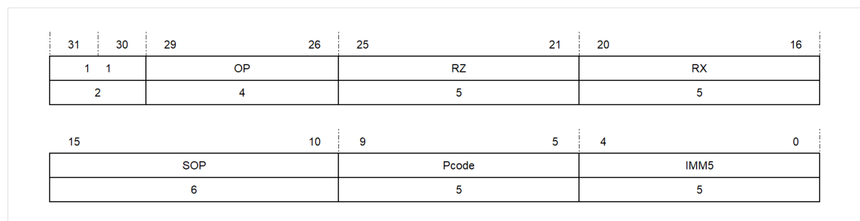
图 4.15: 二元寄存器五位立即数寻址方式第二种格式
