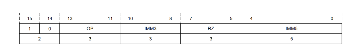
图 5.8: 8 位立即数的编码方式第二种格式
