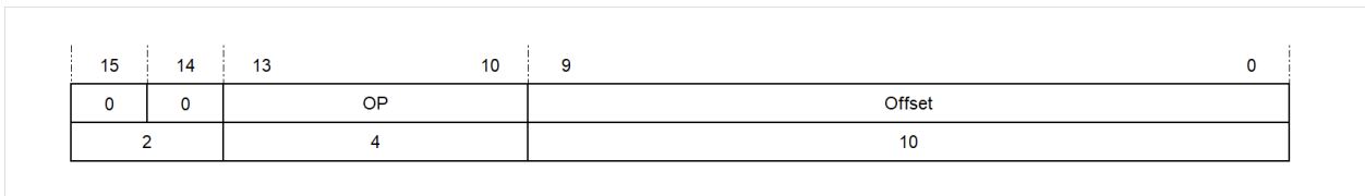
图 5.11: 十位立即数寻址方式
