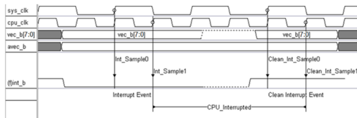
图 7.2: 中断处理过程
