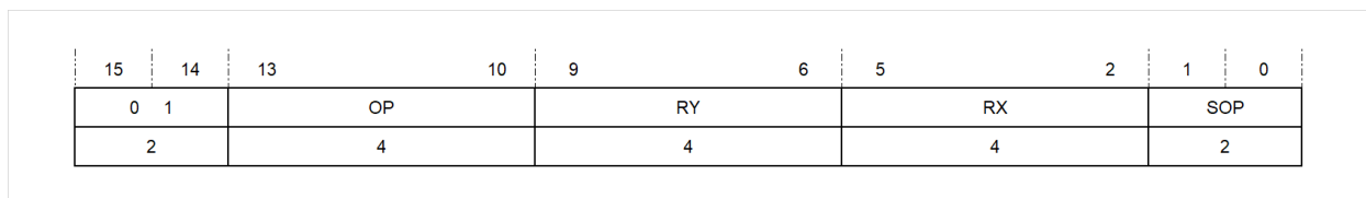
图 5.22: 二元寄存器寻址模式第一种格式
