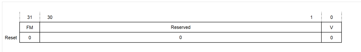
图 3.4: DSP 控制状态寄存器
