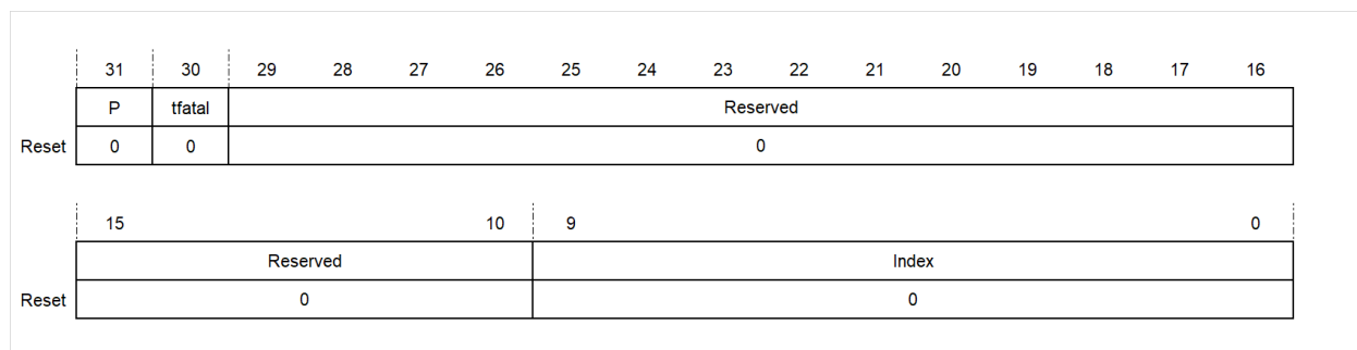
图 3.11: MMU 索引寄存器
